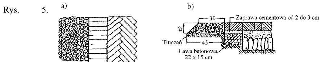
Obramowanie jezdni z klinkieru ułożonego prostopadle do osi drogi
