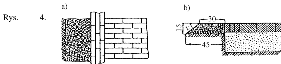
Obramowanie jezdni z trzech rzędów klinkieru z umocowaniem warstwą tłucznia
