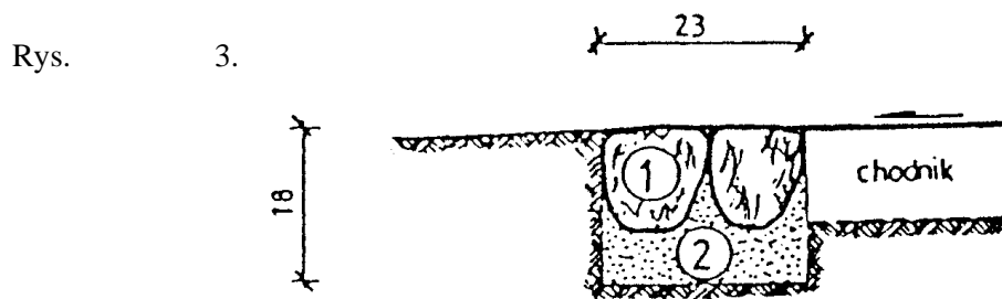
Obramowanie chodnika z brukowca od 10 do 12 cm
